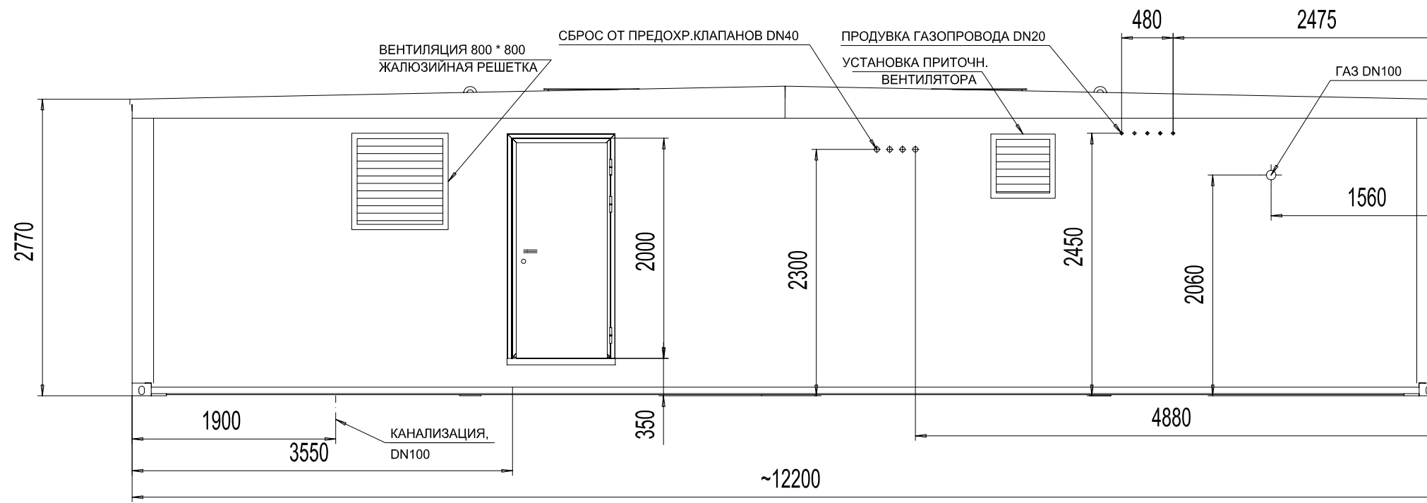
ВИД В
