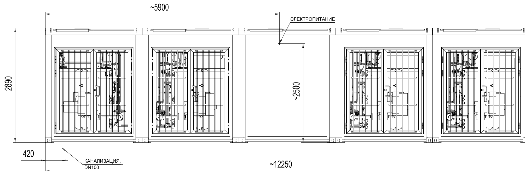
ВИД А
